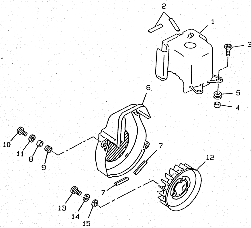
FIG 3 AIR SHROUD. FAN
